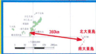
【漁港建設地：北大東地区】
